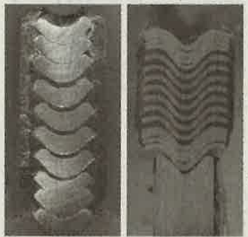
従来品(左)に比べて「チェンジ」は金属板部分が太い(渦巻き型ガスクケットの断面図)
